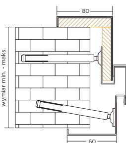
ościeżnica regulowana PU-PR z profilem sprzęgającym
