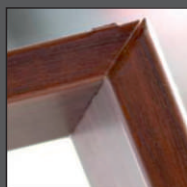
POŁĄCZENIE BELEK OŚCIEŻNICY STALOWEJ PU, PD, PM POD KĄTEM 45°
