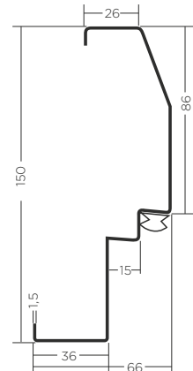
OŚCIEŻNICA PM84/150
