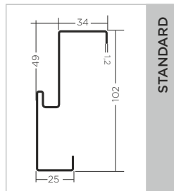
ościeżnica PU68
