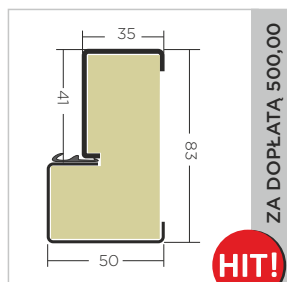
ościeżnica PD56/150
