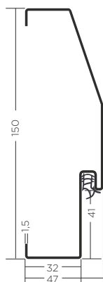
OŚCIEŻNICA PD56/150
