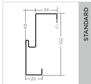
ościeżnica PU68
