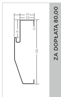
ościeżnica PD56/150
