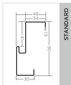
ościeżnica PU56
