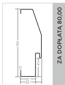
ościeżnica PD56/150
