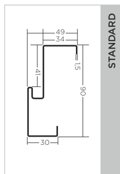
ościeżnica PU56
